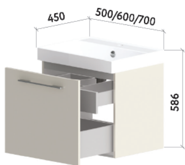
НИЖНИЙ ШКАФ С РАКОВИНОЙ Внутренний ящик
