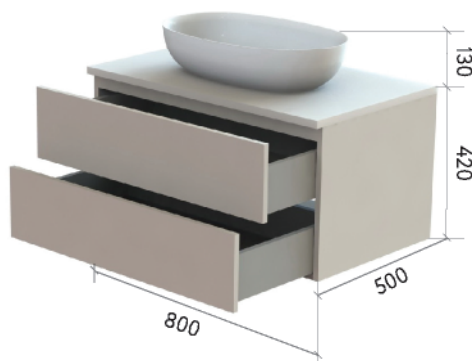
ШКАФ НИЖНИЙ 800-400-1
