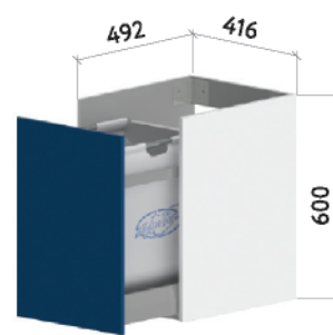
НИЖНИЙ ШКАФ 400 С бельевым мешком
