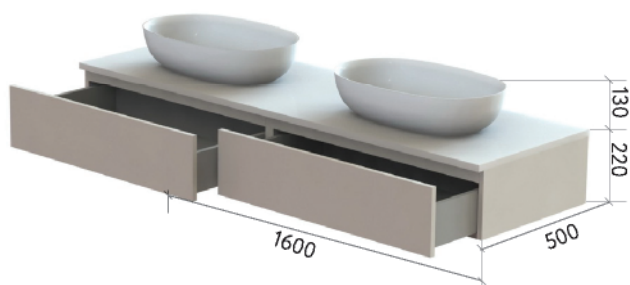
ШКАФ НИЖНИЙ 1600-200-1
