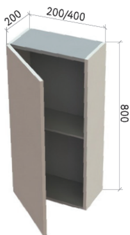
одна полка, 400
