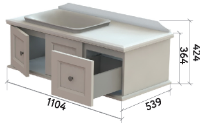
ШКАФ НИЖНИЙ 1100-300-3
