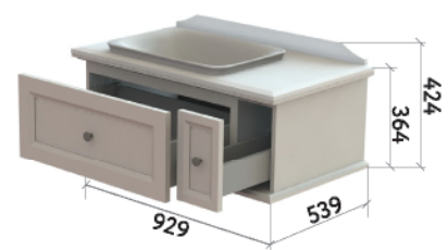
ШКАФ НИЖНИЙ 925-300-2
