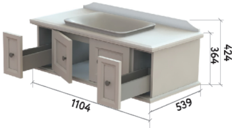
ШКАФ НИЖНИЙ 1100-300-5
