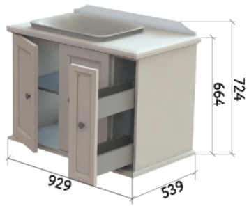
ШКАФ НИЖНИЙ 925-600-1
