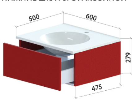
Один ящик, 600
