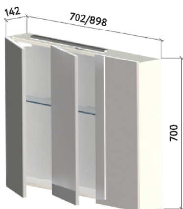
ЗЕРКАЛЬНЫЙ ШКАФ СО СВЕТИЛЬНИКОМ
