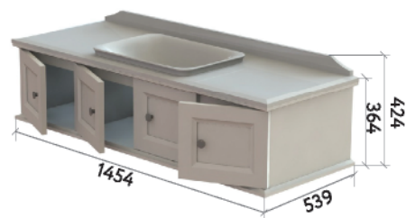
ШКАФ НИЖНИЙ 1450-300-1
