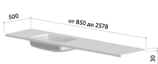
СТОЛЕШНИЦА
