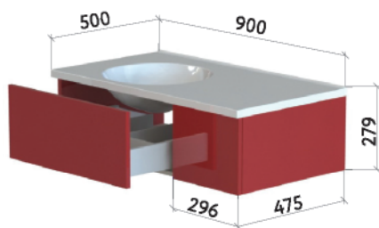
Один ящик, 900
