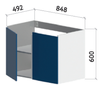
НИЖНИЙ ШКАФ 800 Распашной
