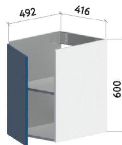
НИЖНИЙ ШКАФ 400 Распашной
