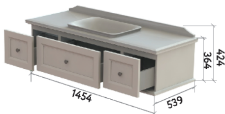
ШКАФ НИЖНИЙ 1450-300-6
