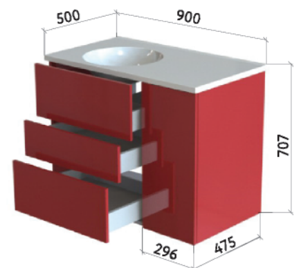
Три ящика, 900
