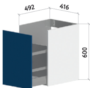
НИЖНИЙ ШКАФ 400 Выдвижной
