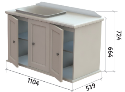
ШКАФ НИЖНИЙ 1100-600-1
