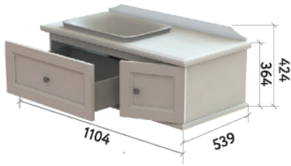
ШКАФ НИЖНИЙ 1100-300-2
