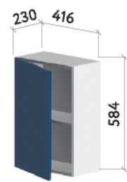
ВЕРХНИЙ ШКАФ 400
