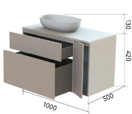
ШКАФ НИЖНИЙ 1000-600-2
