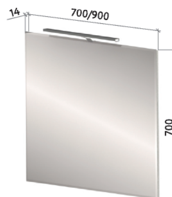
ЗЕРКАЛО
