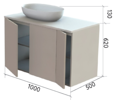
ШКАФ НИЖНИЙ 1000-600-1
