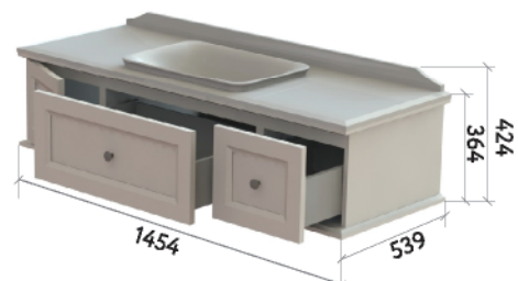
ШКАФ НИЖНИЙ 1450-300-4
