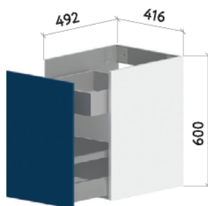
НИЖНИЙ ШКАФ 400 Выдвижной двойной
