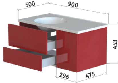
Два ящика, 900
