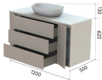
ШКАФ НИЖНИЙ 1200-600-3
