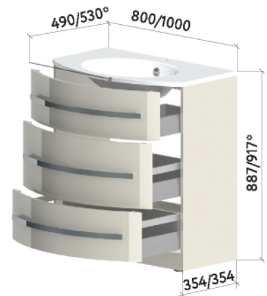
НИЖНИЙ НАПОЛЬНЫЙ ШКАФ С РАКОВИНОЙ Три ящика
