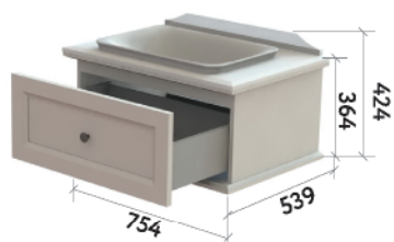
ШКАФ НИЖНИЙ 750-300-2
