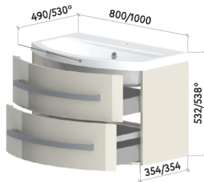
НИЖНИЙ ШКАФ С РАКОВИНОЙ Два ящика
