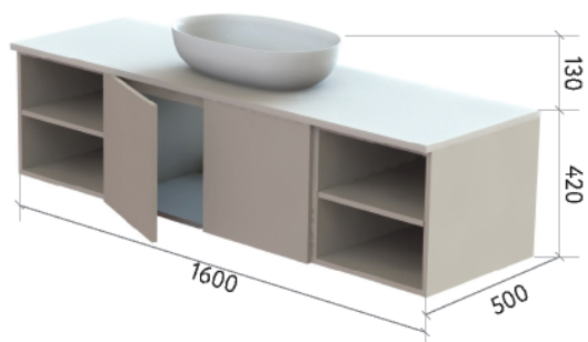
ШКАФ НИЖНИЙ 1600-400-2
