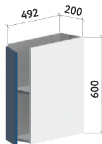
НИЖНИЙ ШКАФ 200 Распашной
