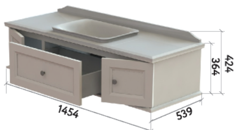
ШКАФ НИЖНИЙ 1450-300-2
