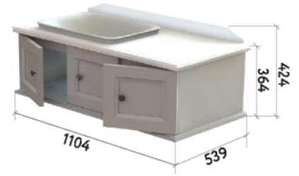
ШКАФ НИЖНИЙ 1100-300-1
