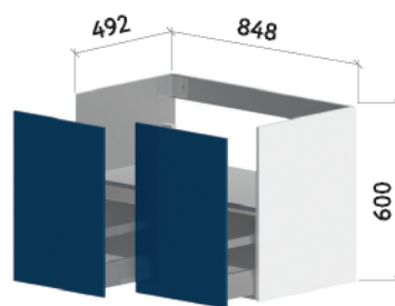
НИЖНИЙ ШКАФ 800 Выдвижной
