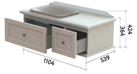
ШКАФ НИЖНИЙ 1100-300-4
