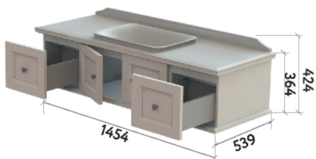
ШКАФ НИЖНИЙ 1450-300-5
