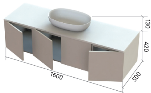
ШКАФ НИЖНИЙ 1600-400-1
